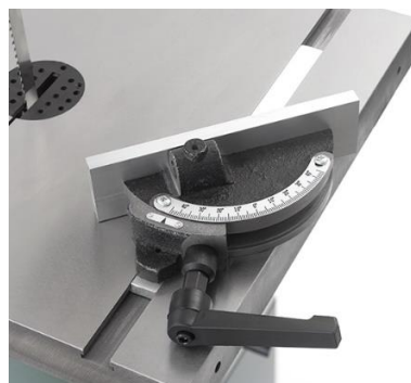
68051 - öntöttvas nehéz vezetővonalzó Sabre szalagfűrészekhez
